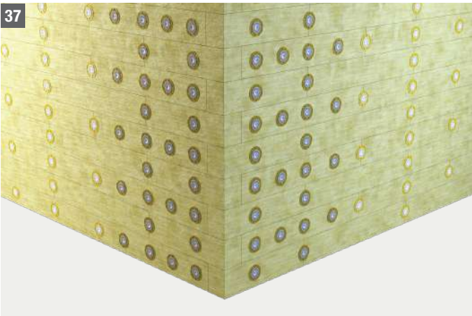
Befestigungsschema für MW-Lamellen (120×20 cm), an der Oberfläche 6 Befestigungselemente und in der Randzone 12
