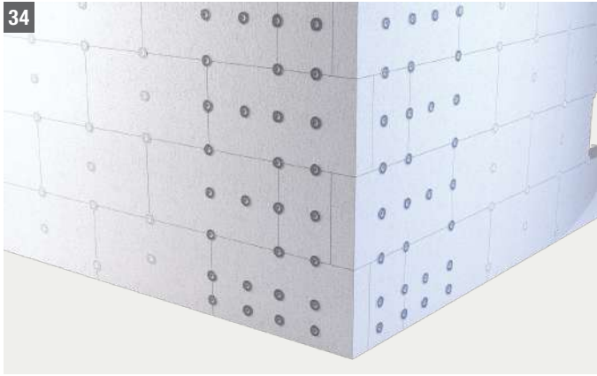
T-Schema 6 Dübel an der Oberfläche und Randzone mit 12 Dübeln für EPS F-Platten (100×50 cm)
