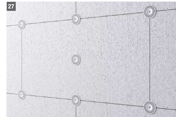
T-Schema 6 Befestigungselemente für EPS F-Platten (100×50 cm)
