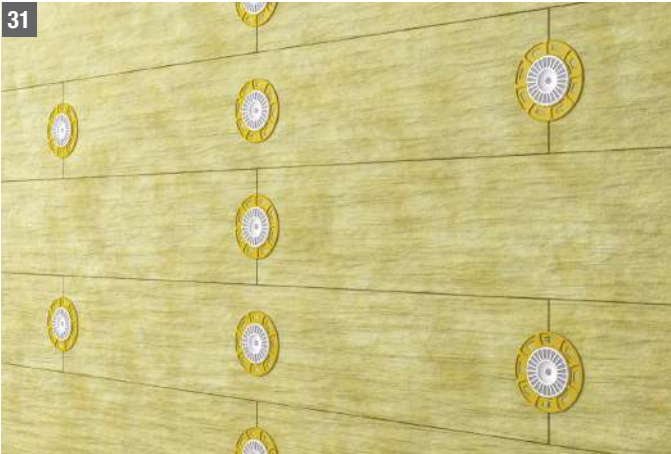
Schema Befestigungselemente für MW-Lamellen (120×20 cm)
