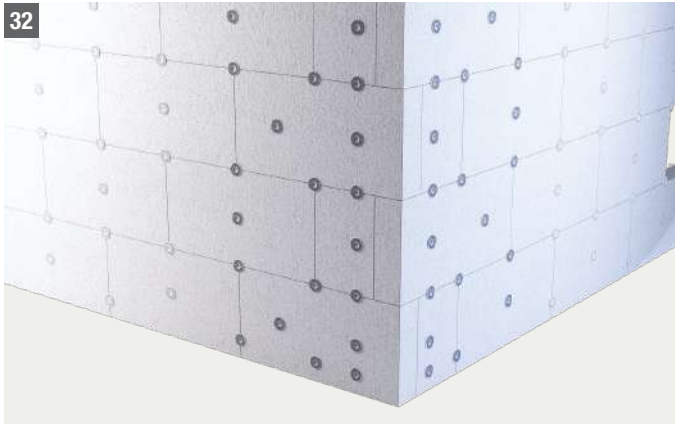
T-Schema 6 Dübel an der Oberfläche und Randzone mit 10 Dübeln für EPS F-Platten (100×50 cm)
