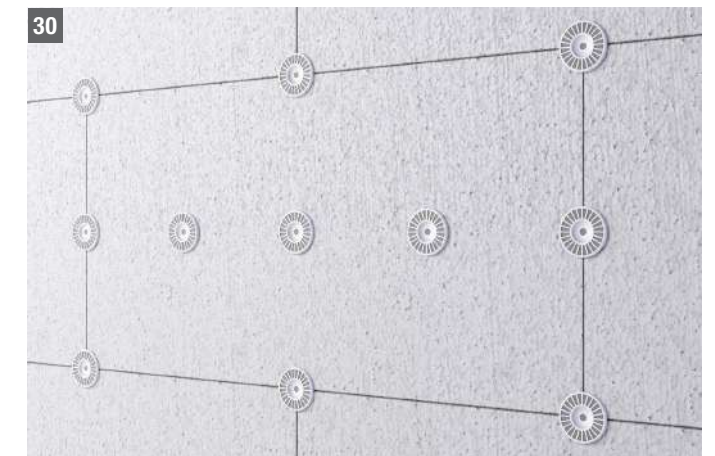
T-Schema 12 Befestigungselemente für EPS F-Platten (100×50 cm)
