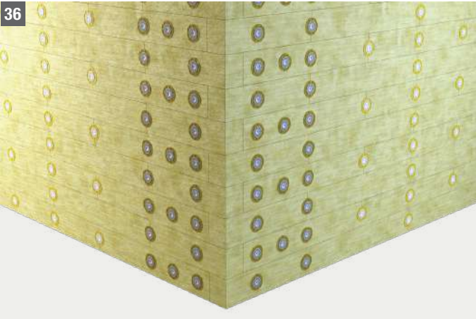
Befestigungsschema für MW-Lamellen (120×20 cm), an der Oberfläche 6 Befestigungselemente und in der Randzone 10
