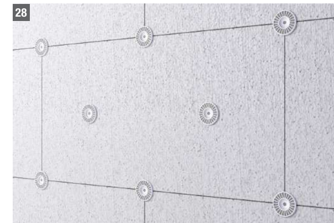
T-Schema 8 Befestigungselemente für EPS F-Platten (100×50 cm)
